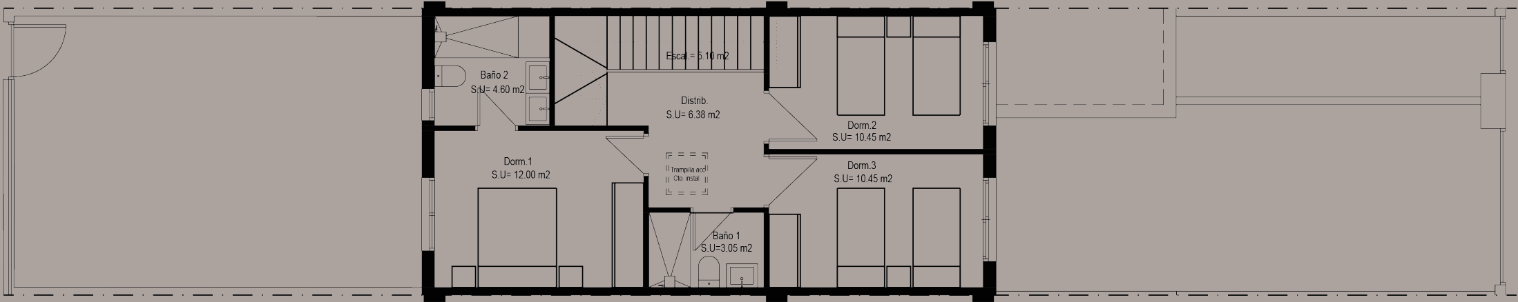
PLANTA PRIMERA
