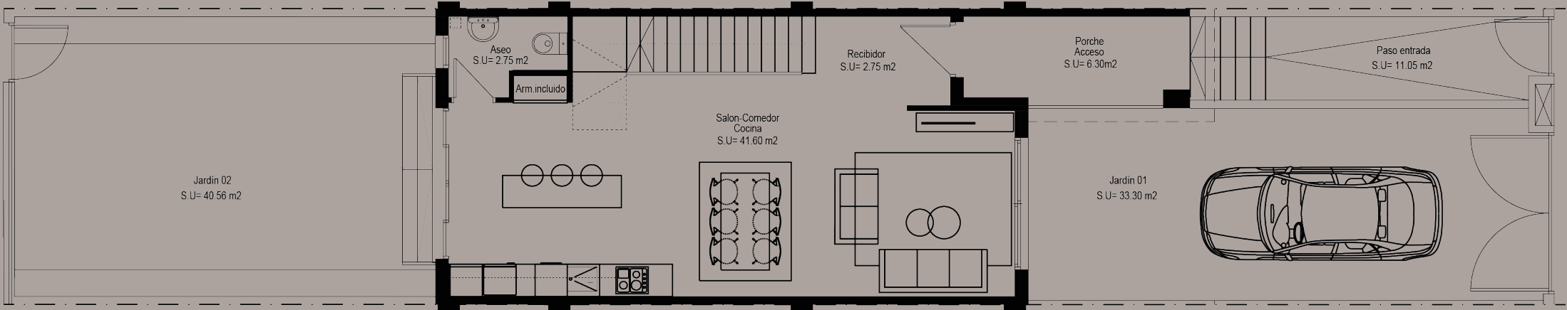
PLANTA BAJA
